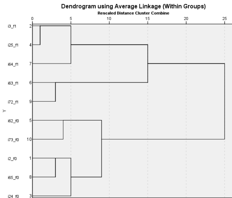
Фигура 4: Дендрограма от полярни убеждения с Pearson's correlation method
