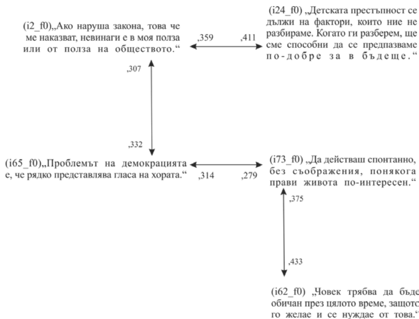
Фигура 6: Диаграма на пътеките между хуманистичните убеждения
