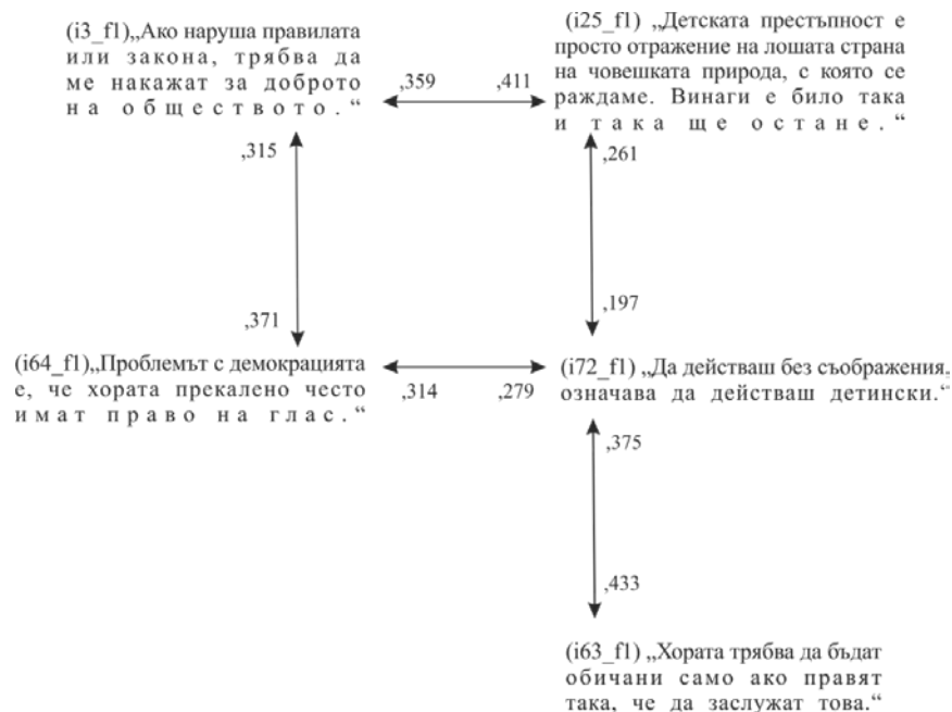
Фигура 5: Диаграма на пътеките между нормативистичните убеждения
